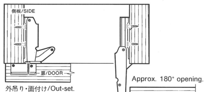
■ 平面図/PLAN
