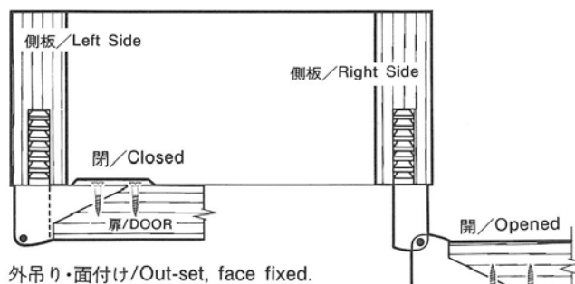
■ 平面図/PLAN
