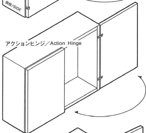
K. 広角アクションヒンジ/Action Hinge
