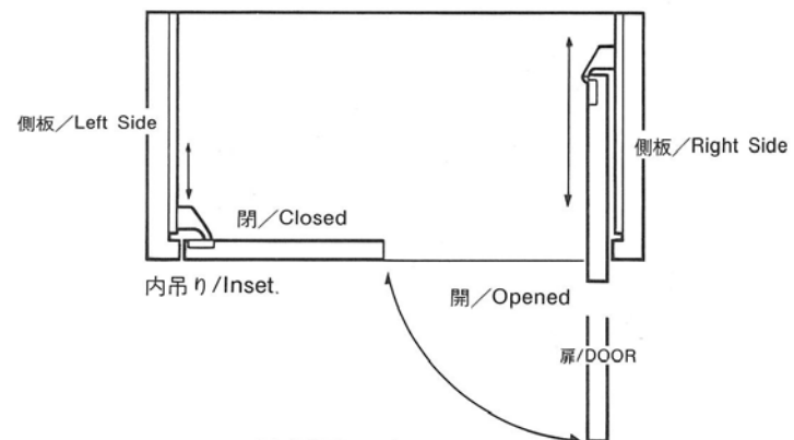
■ 平面図/PLAN
